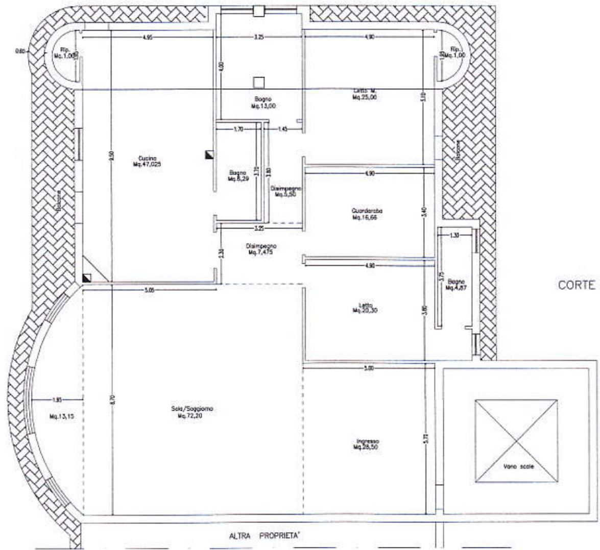
PIANTA QUOTATA PIANO SECONDO Sup. Lorda mq.287,31 Sup. Utile Abitabile mq.260,97
